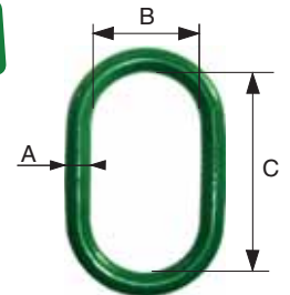
ANNEAU SIMPLE ref. 5058 Pour élingues-câble 1 et 2 brins
