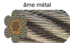
6 x 36 fils
